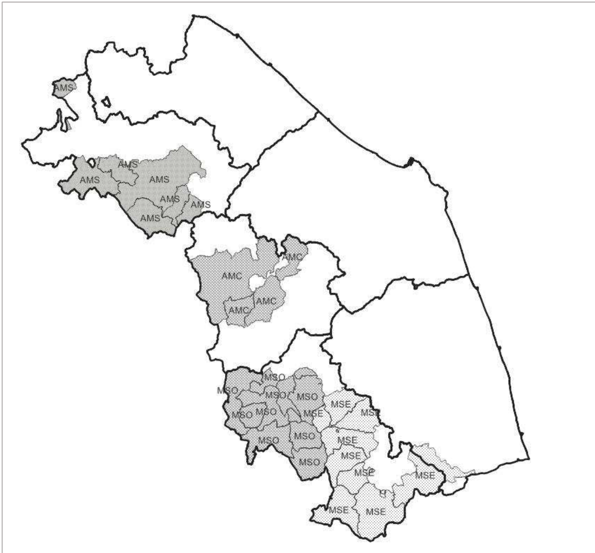
Figura 3. Zone di allerta per il rischio valanghe
