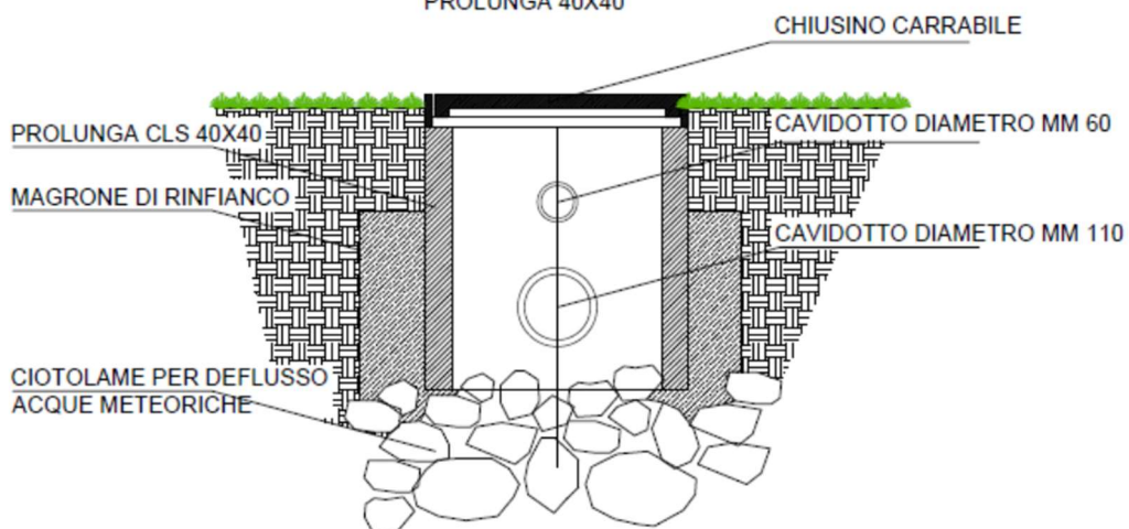
PARTICOLARE POZZETTO DI DERIVAZIONE LINEE ELETTRICHE E SEGNALI LUCI PERIMETRALI PROLUNGA 40X40
