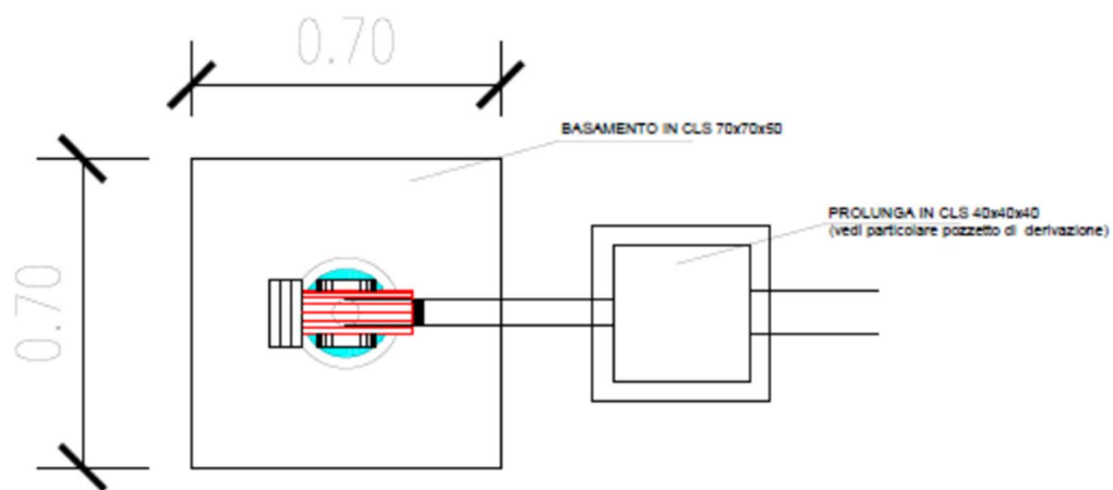
PARTICOLARE BASAMENTO INDICATORE DELL'ANGOLO DI PLANATA GPI
