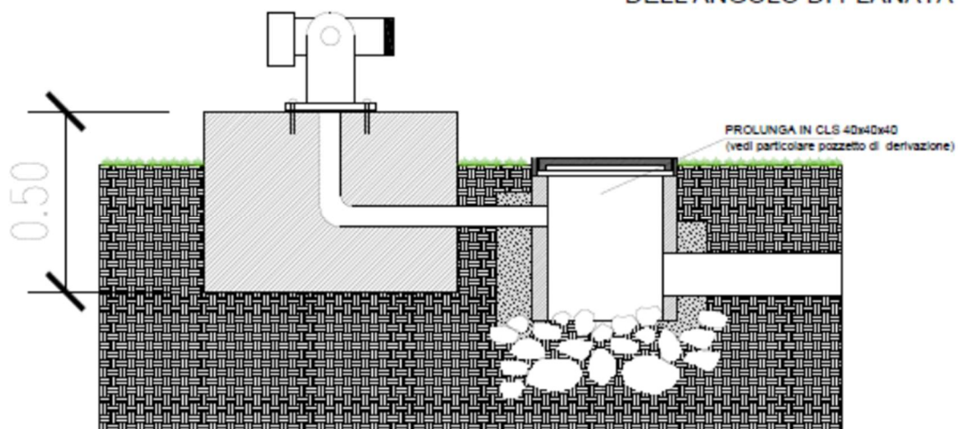
PARTICOLARE POZZETTO DI DERIVAZIONE LINEE ELETTRICHE E SEGNALI LUCI PERIMETRALI PROLUNGA 40X40
