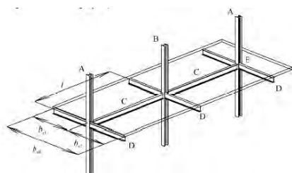
Fig. 7.6.2 - Definizione degli elementi in una struttura intelaiata
