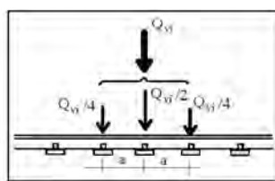
Fig. 5.2.3 - Distribuzione longitudinale dei carichi assiali
