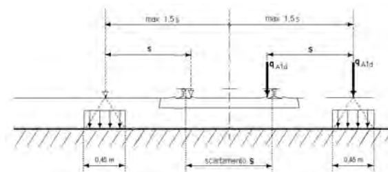
Fig. 5.2.12 - Caso 1
